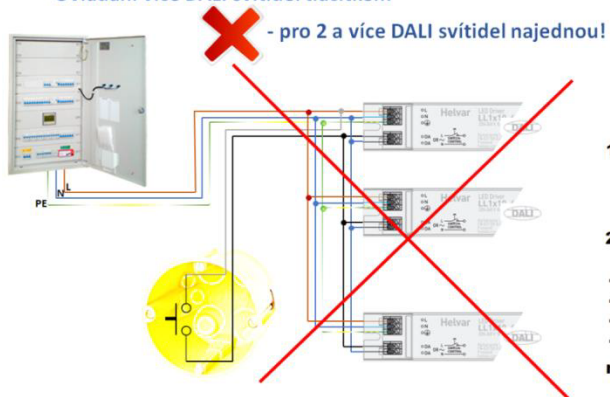
Ovládání více DALI svítidel tlačítkem
