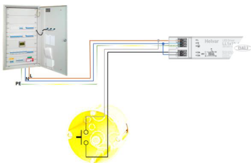
Ovládání jednoho DALI svítidla tlačítkem pomocí fáze
